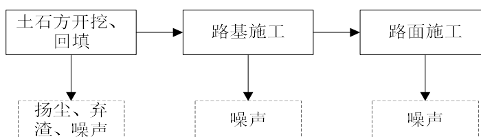
图 2-4 进场道路施工工艺流程及产污节点图
