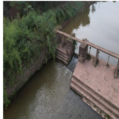
冲沙孔现状
