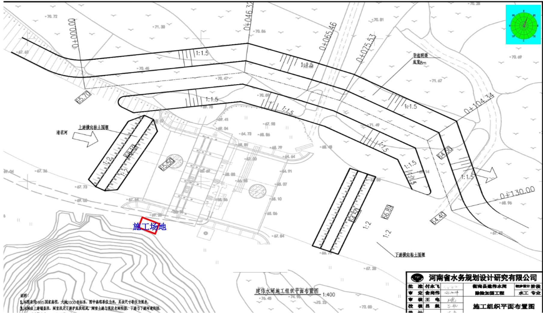
附图3 项目施工总平面布置图
