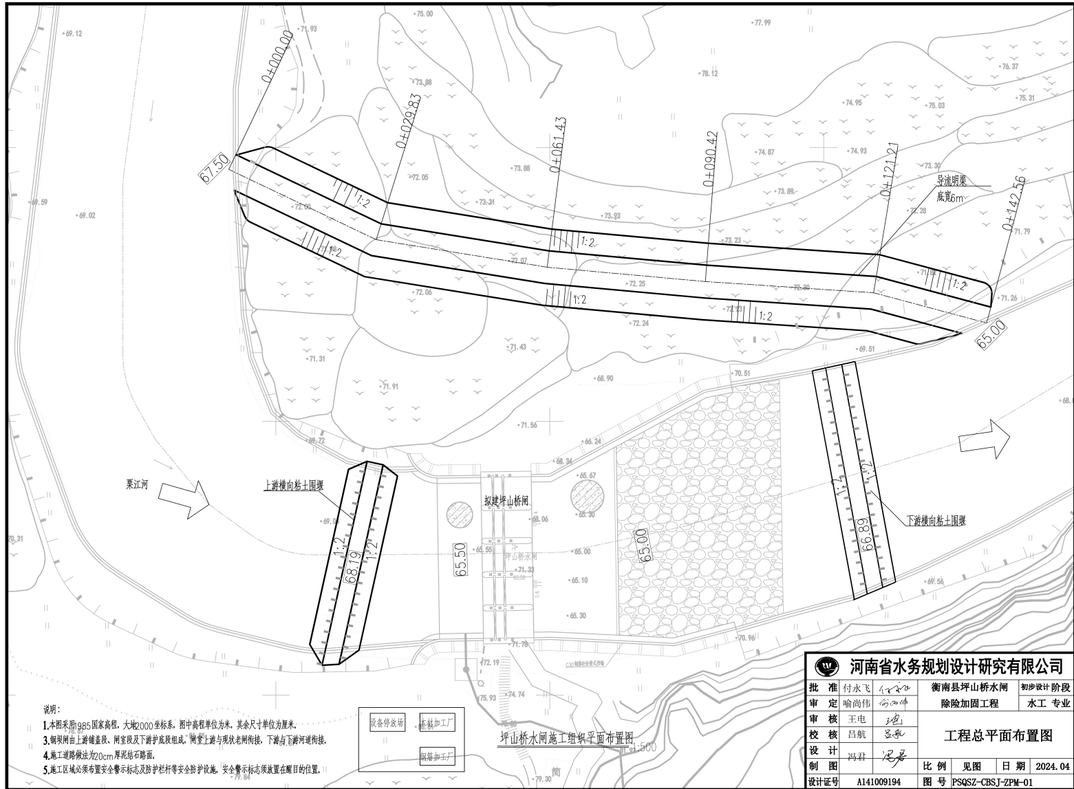
附图3 项目施工总平面布置图
