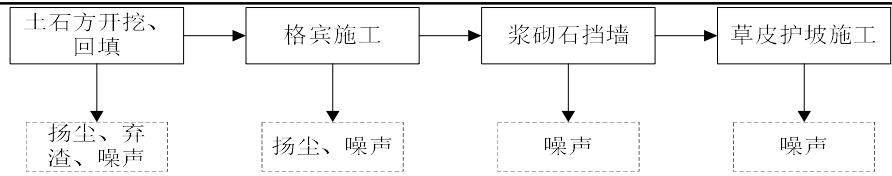
图 2-3 护岸工程施工工艺流程及产污节点图
