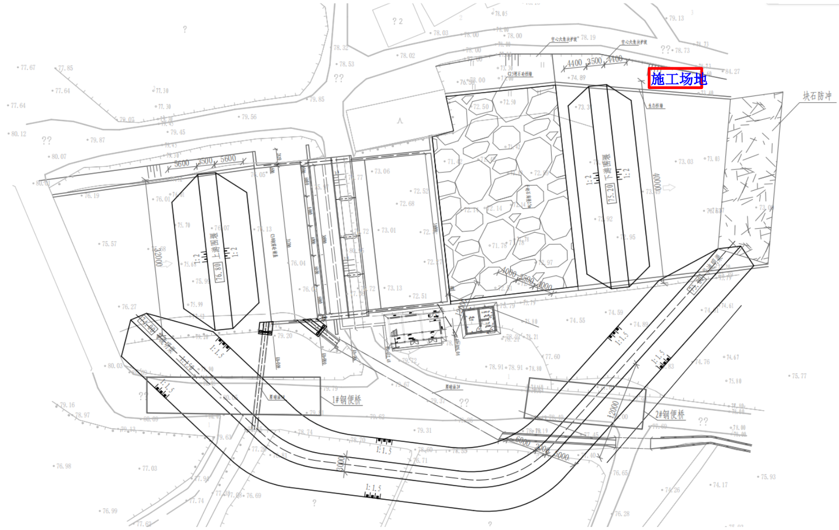
附图3 项目施工总平面布置图
