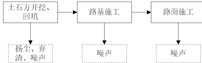
图 2-5 进场道路施工工艺流程及产污节点图
