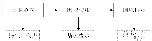
图 2-1 围堰施工工艺流程及产污节点图
